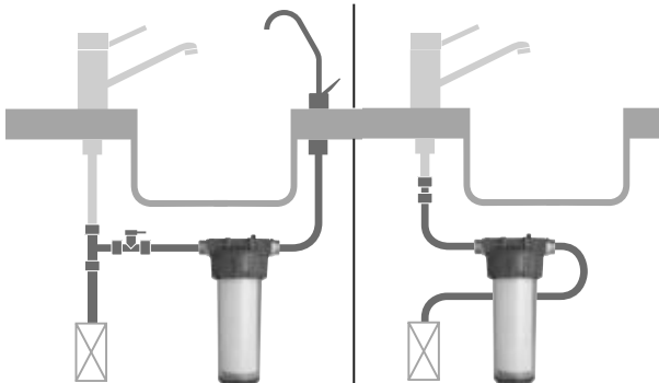
Einbauschema VARIO Classic & Comfort VARIO Küche ohne Hahn
